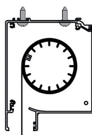
FISSAGGIO CON VITE DIRETTA A SOFFITTO
