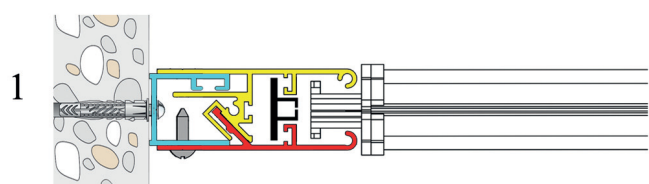
GUIDA ZIPPY A FISSAGGIO LATERALE, REGOLABILE PER FUORISQUADRO DA 63 A 78MM
