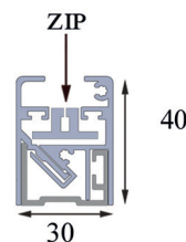
GUIDA ZIPPY SLIM A FISSAGGIO LATERALE, REGOLABILE PER FUORISQUADRO DA 40 A 48MM
