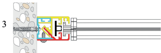
GUIDA ZIPPY SLIM A FISSAGGIO LATERALE, REGOLABILE PER FUORISQUADRO DA 40 A 48MM
