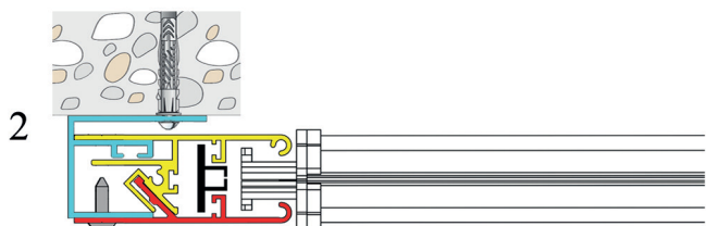
GUIDA ZIPPY A FISSAGGIO FRONTALE, REGOLABILE PER FUORISQUADRO DA 65 A 80MM
